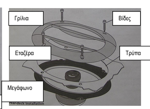
Παράδειγμα τοποθέτησης ηχείου σε εταζέρα
